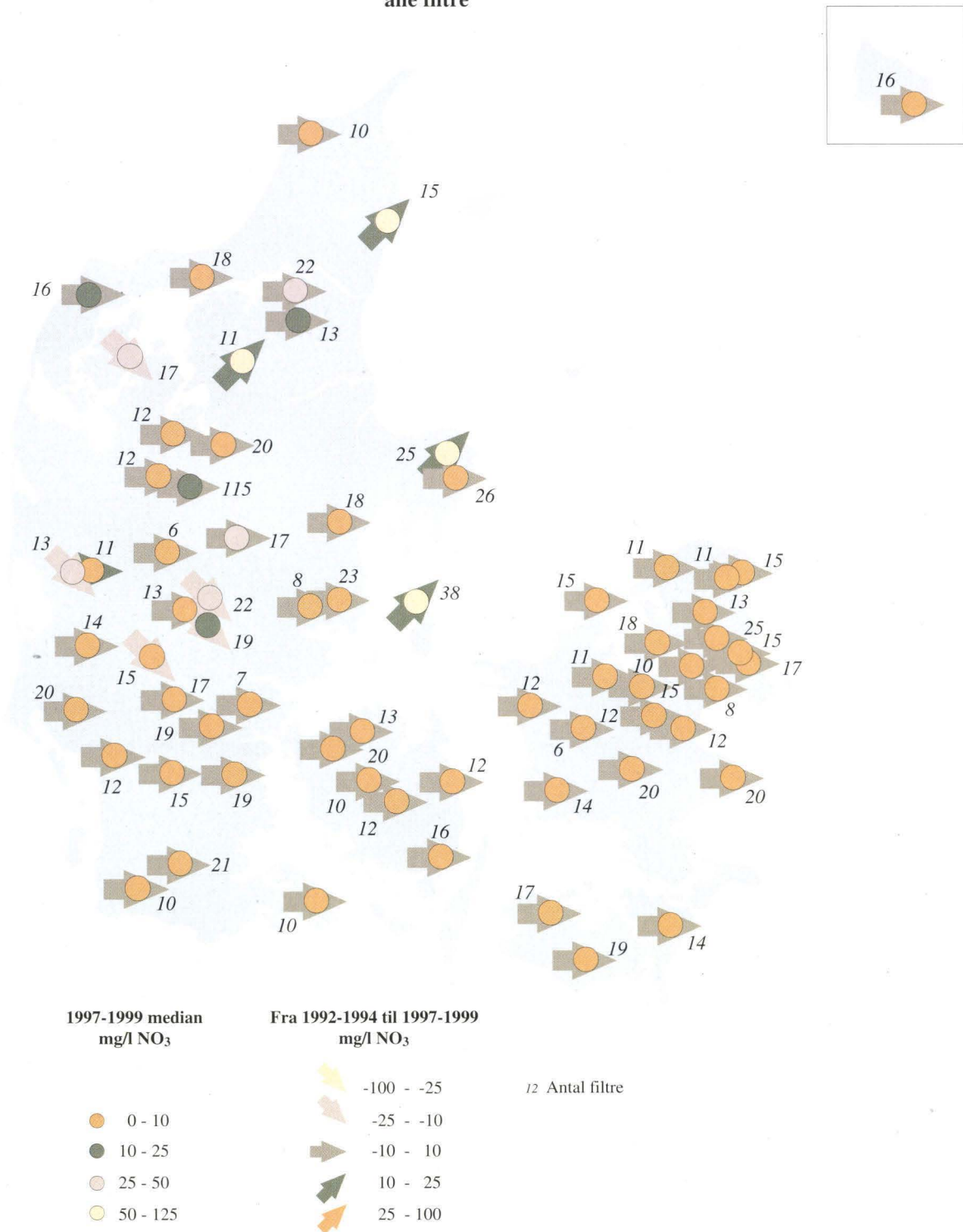
Figur 2.6 Nitratindhold og -udvikling baseret på alle nitratdata i GRUMO (Nyegaard & Stockmarr 2000).
