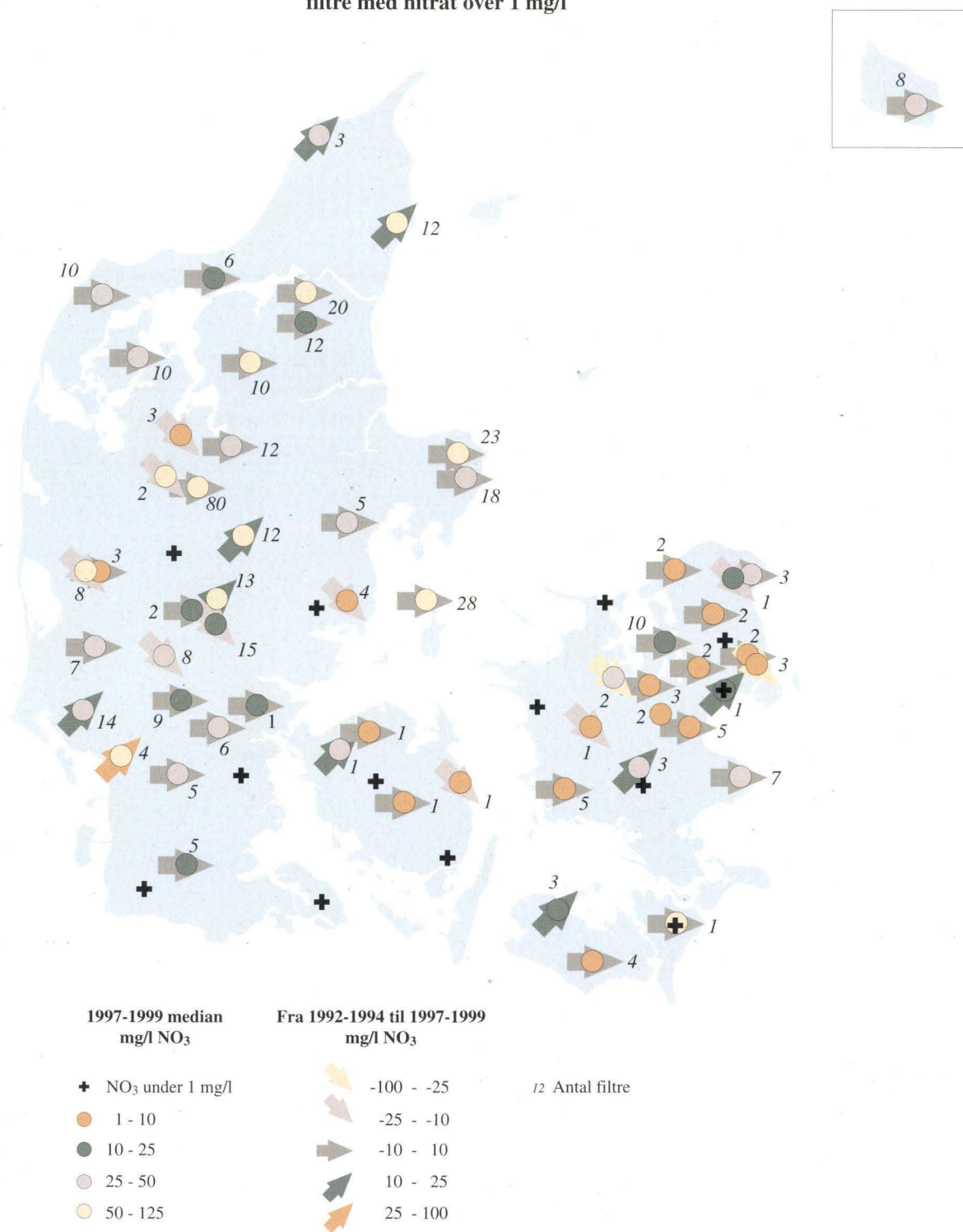
Figur 2.7 Nitratindhold og -udvikling baseret på nitratdata over 1 mg/l i GRUMO (Nyegaard & Stockmarr 2000).
