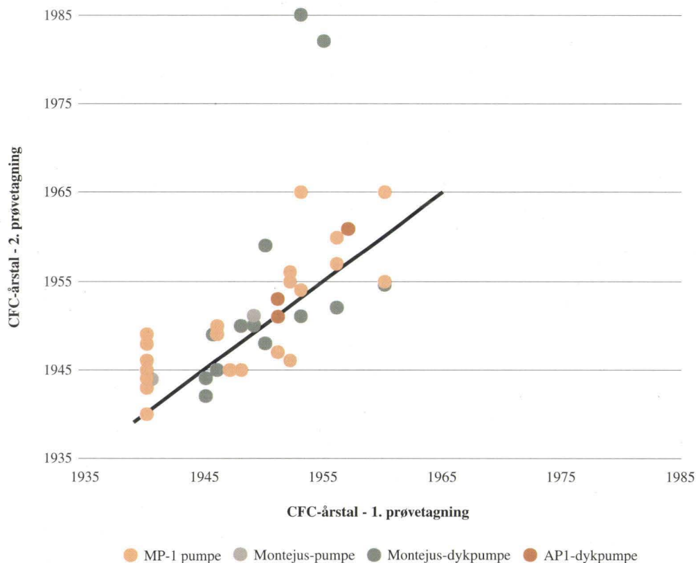
Figur 8.3. Sammenligning af CFC-resultaterne af 1. og 2. prøvetagning. Tidsrummet mellem de to prøvetagninger var 1-1½ år.
